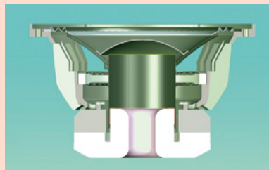
Aufbau, Schnittbild und Magnetfeldsimulation des Mitteltöners von JBLs Summit Makalu und Pumori: Neodym-Antrieb mit belüftetem Polkern, Faraday-Ring und Alu-Schwingspule reduzieren Verzerrungen. Doppelte Zentrierspinne, Carbon-Sandwichmembran und große Kalotte sorgen für Kontrolle und Dynamik.
