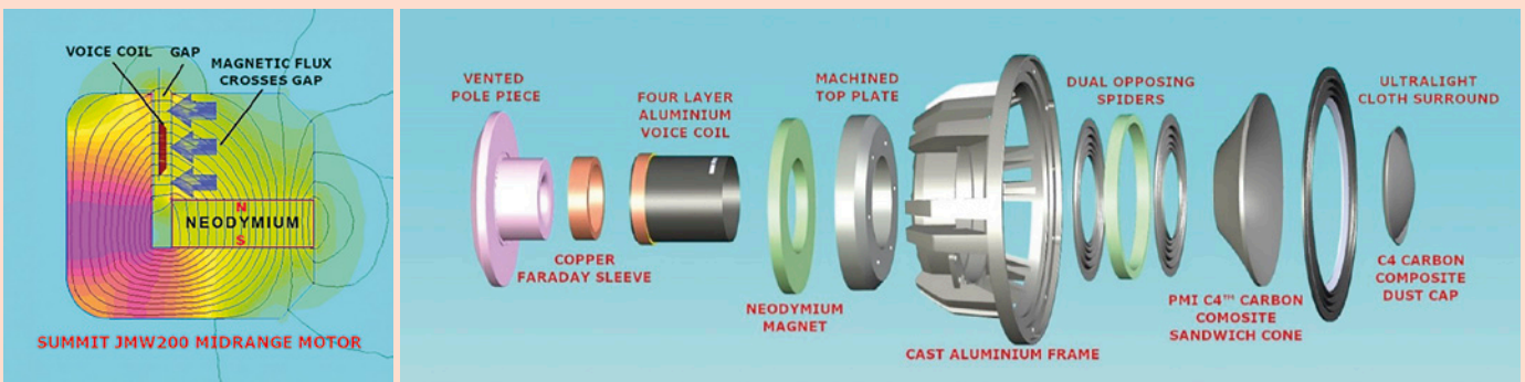
Aufbau, Schnittbild und Magnetfeldsimulation des Mitteltöners von JBLs Summit Makalu und Pumori: Neodym-Antrieb mit belüftetem Polkern, Faraday-Ring und Alu-Schwingspule reduzieren Verzerrungen. Doppelte Zentrierspinne, Carbon-Sandwichmembran und große Kalotte sorgen für Kontrolle und Dynamik.
